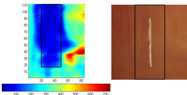
Figure 2 : cartographie (60/70mm) de potentiel (en volt) et photographie du revêtement
