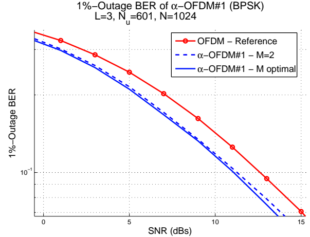
Fig. 3. \alpha -OFDM#1 BER
