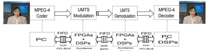
Fig. 19. MPEG-4 over UMTS FDD.
