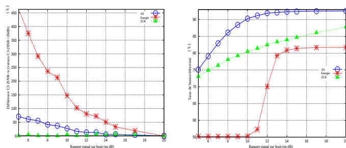
FIG. 6 – Gauche : Différence en % de la valeur de C_3 apprise pour différents SNR, la valeur obtenue pour un SNR de 20 dB étant prise comme référence ; Droite : TBD, pour différents SNR, C_3 pas ajusté au SNR ; T = 14 ms
