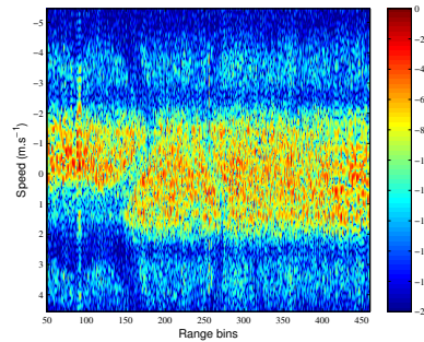
Figure 10. Carte Doppler-distance d'un des capteurs
