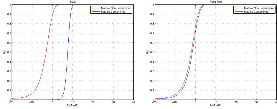
Figure 6. Performances de détection ( P_{fa}=0.01 ) d'une cible pour une cellule de référence fortement contaminée (20 dB) ou pas. a) gauche, performances de l'AMF avec SCM biaisée ou pas par la contamination. b) droite, performances de l'ANMF avec l'estimateur robuste du point fixe
