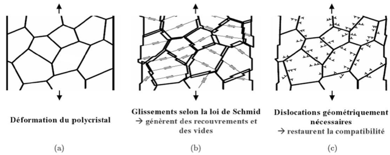
Figure 3.1. Représentation de la déformation plastique d'un polycristal d'après Ashby
