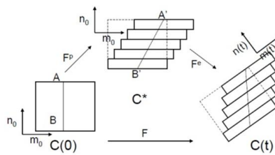
Figure 3.10 : Schéma représentant la décomposition de la transformation \tilde{F} = \tilde{F}^e \tilde{F}^p
