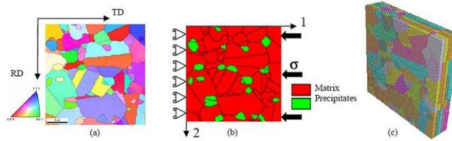
Figure 3.22 : (a) carte d'orientations de l'agrégat extrudé. (b) Conditions aux limites imposées et visualisation des deux phases. (c) Agrégat formé de 4 couches identiques [THE 08].
