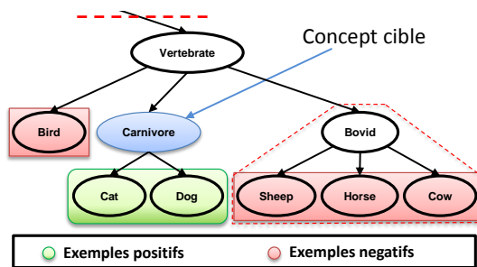
Figure 5. Apprentissage des classifieurs hiérarchiques «un-contre-nœuds-opposés»
