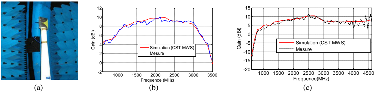
Figure 4. (a) Système de mesure sphérique de Supélec, (b) Gain réalisé pour l'antenne Vivaldi, (c) Gain réalisé pour l'antenne spirale.
