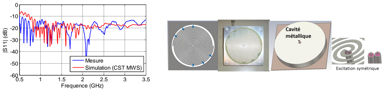
Figure 1. (à gauche) Comparaison des données de simulation et de mesure du S_{11} de l'antenne spirale. (à droite) antenne spirale en présence des charges résistives (flèches bleues), la cavité métallique sous l'antenne et le système d'excitation utilisé pour l'antenne spirale.
