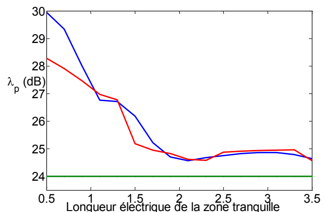
Figure 2. Contraste de pic dans la zone tranquille en fonction de la longueur électrique L_e ; courbe bleue et rouge respectivement avec et sans optimisation, courbe verte contraste de pic requis pour le mesure [3].
