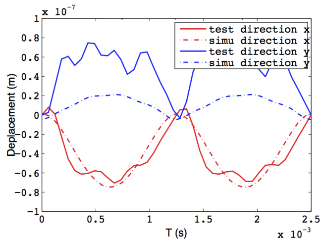
FIGURE 2 – Exemple de comparaison modèle/essai : déplacement horizontal (x) et vertical (y) du coin inférieur gauche - f=400\text{Hz} , i=50\text{A} .tours.
