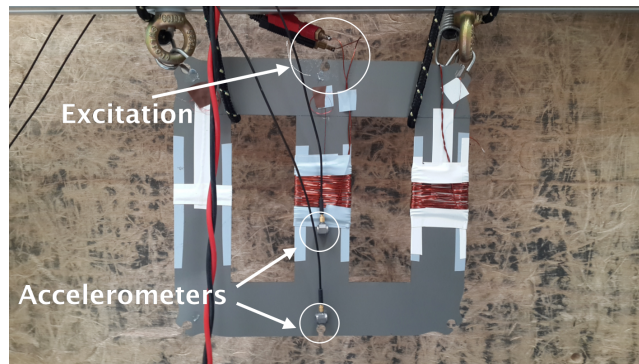
FIGURE 1 – Banc de mesure expérimental.
