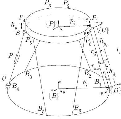
Fig. 1. Stewart-Gough robot.
