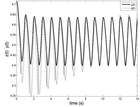
Fig. 1. Input signal.
