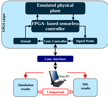
Fig. 16. HIL procedure
