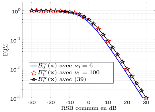
FIGURE 2 – Expressions des bornes asymptotiques pour deux modèles ( M_0 ) et ( M_1 ) à RSB fixé.
