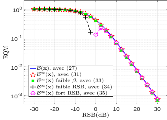
FIGURE 1 – \mathcal{B}(\mathbf{x}) en fonction du RSB en dB avec les approximations correspondant aux régimes limites de la section 4.2.1.
