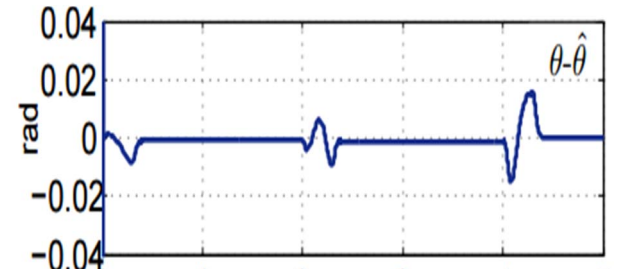
d. Rotor position estimation error
