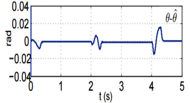
d. Rotor position estimation error
