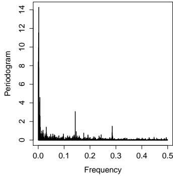
(c) Robust periodogram.
