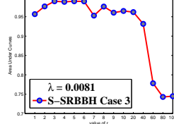
Fig. 3. AUCs: Case 3
