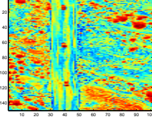
Fig. 2. DATA (average)
