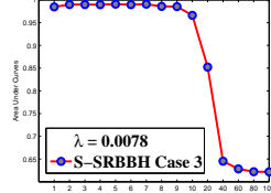
Fig. 8. AUCs: Case 3
