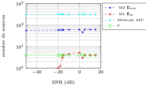
FIGURE 3 – Estimation de p (4 tirages), m = 400 , c = 0.2 , p = 4 sources, en fonction du SNR.
