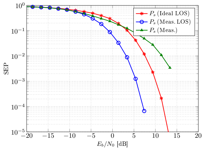
(d) Scenario I, 4 \times 4 MIMO with \eta = 4
