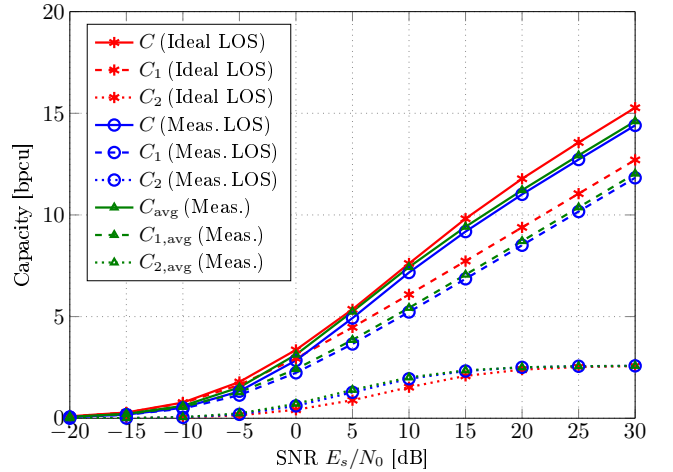
(d) Scenario I, 4 \times 4 MIMO with \eta = 4
