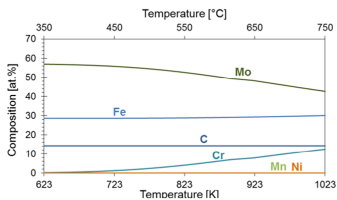
Fig. 11b – M_6C
