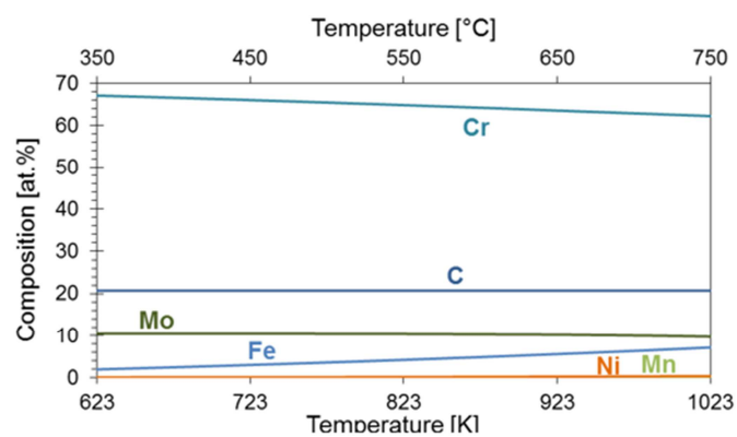
Fig. 11c – M_{23}C_6
