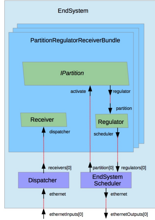
Fig. 3. A664 EndSystem
