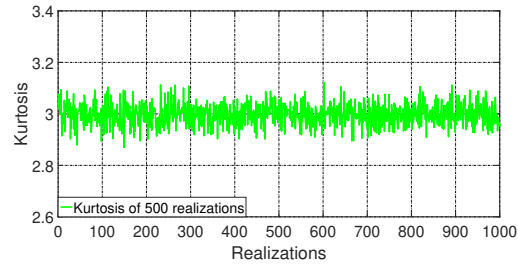
(d) Kurtosis ( R_{sc} = 100\Omega )
