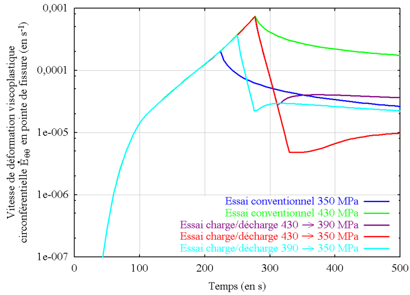
(a) Vitesse de déformation viscoplastique circonférentielle \dot{E}_{\theta\theta}^{vp} .
