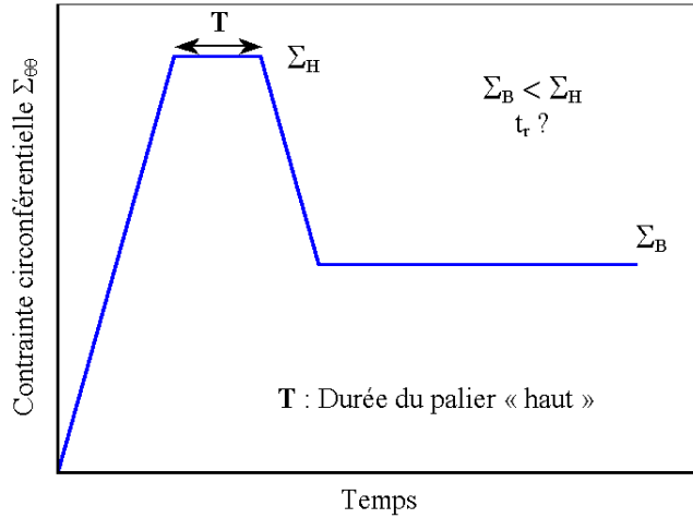
FIG. VI-4. Description de l'essai de « charge/décharge ».
