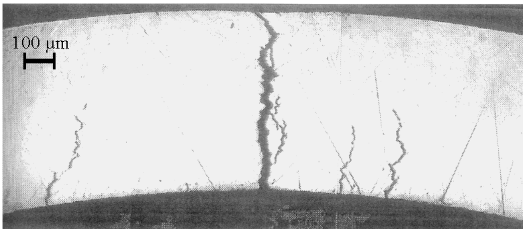
FIG. II-3. Exemple de crayon rompu montrant la faible réduction d'épaisseur de la gaine au niveau de la fissure débouchante [Boyer et al. 1994].
