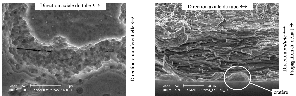
FIG. VII-11. Localisation des sites d'amorçage dans le Zircaloy-4 détendu. Essais conventionnels de CSC ( \Sigma_{\theta\theta} = 350 MPa) réalisés à la température de 350 °C.
