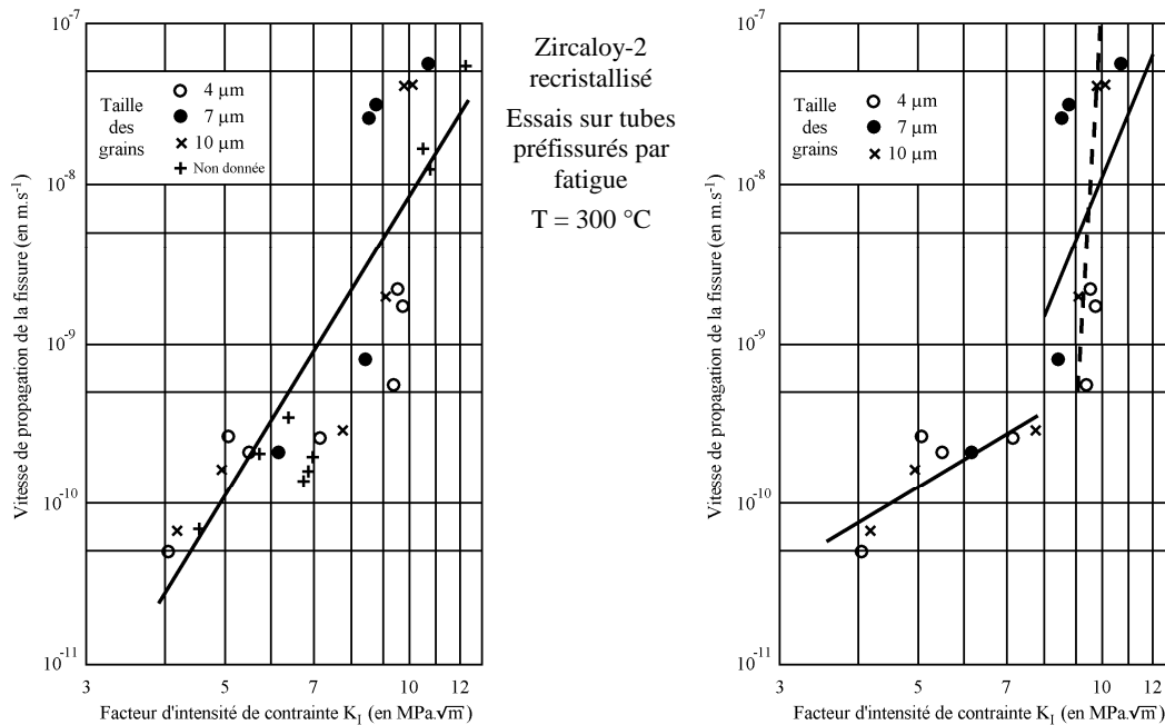
FIG. III-14. Vitesse de propagation d'une fissure de CSC en fonction de K_I [Norrington et al. 1982].
