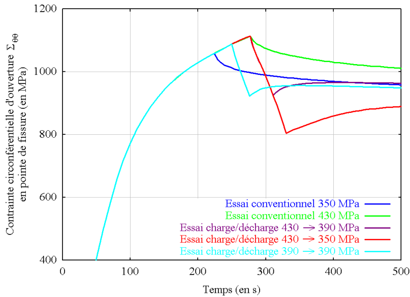
(b) Contrainte circonférentielle d'ouverture de la fissure \Sigma_{\theta\theta} .
