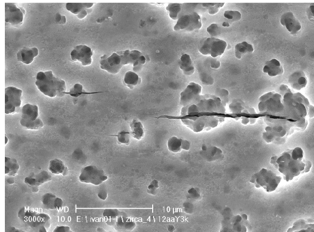
(c) Essai conduit à rupture (3,4 heures)
