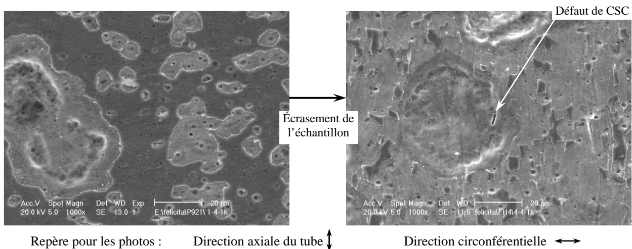
FIG. VII-5. Desquamation de la couche d'oxyde suite à l'écrasement de l'échantillon (essai de CSC conventionnel, \Sigma_{\theta\theta} = 350\ \text{MPa} , durée de vie de 5,6 heures).
