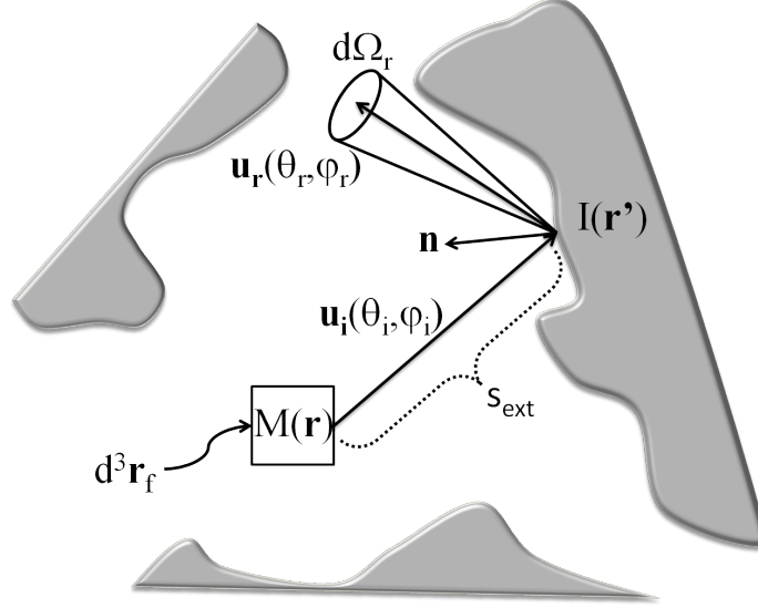
FIGURE 2.7 – Représentation schématique de l'étape de lancer de rayon de l'algorithme de Monte Carlo pour la caractérisation des propriétés radiatives.
