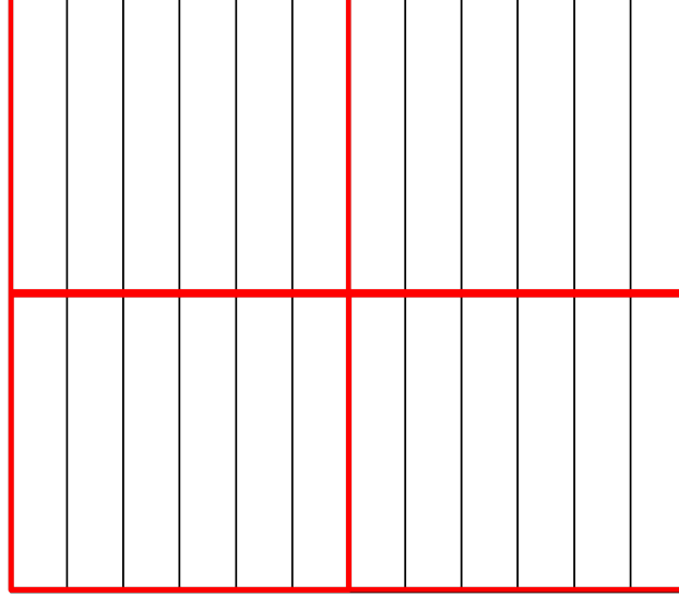
FIGURE 2.6 — En 2D, 4 zones délimitées par les traits rouges sont représentées. Ces zones peuvent contenir plusieurs particules ; les volumes élémentaires, délimités par des traits noirs, sont eux petits par rapport à la taille des particules. Les zones n'ont pas d'autre utilité que de diminuer les temps de calcul lorsque l'empilement est de grande taille.
