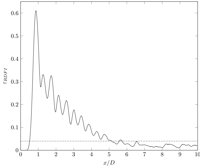
FIGURE 3.19 – Empilement A : valeur du critère \varepsilon_{RDFI}(x, \mathbf{u}) pour \mathbf{u} = -\mathbf{x} (courbe noire) et limite de validité \varepsilon_{RDFI}(x, \mathbf{u}) = 4\% (courbe pointillée).
