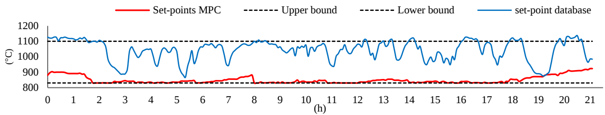
Fig. 33 : Consignes de température de zone préchauffe
