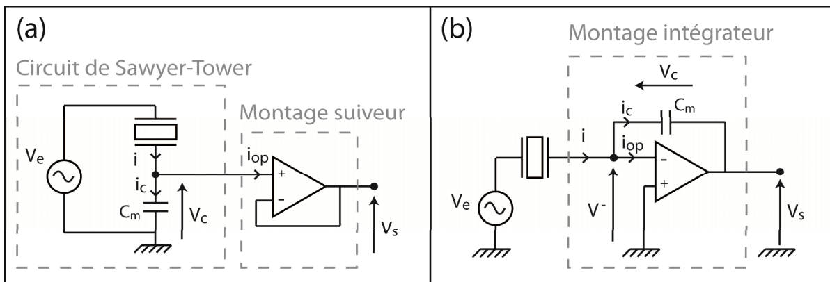
Figure 4-1 : Circuit de Sawyer-Tower suivi d'un montage suiveur (a) et montage intégrateur (b).
