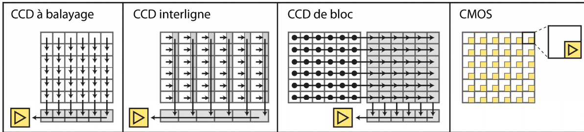
Figure 3-4 : Représentation d'un capteur CCD dans le cas d'un transfert à balayage (a), interligne (b) et de bloc (c). Représentation d'un capteur CMOS (d). Les illustrations ont été réalisées d'après [178] .
