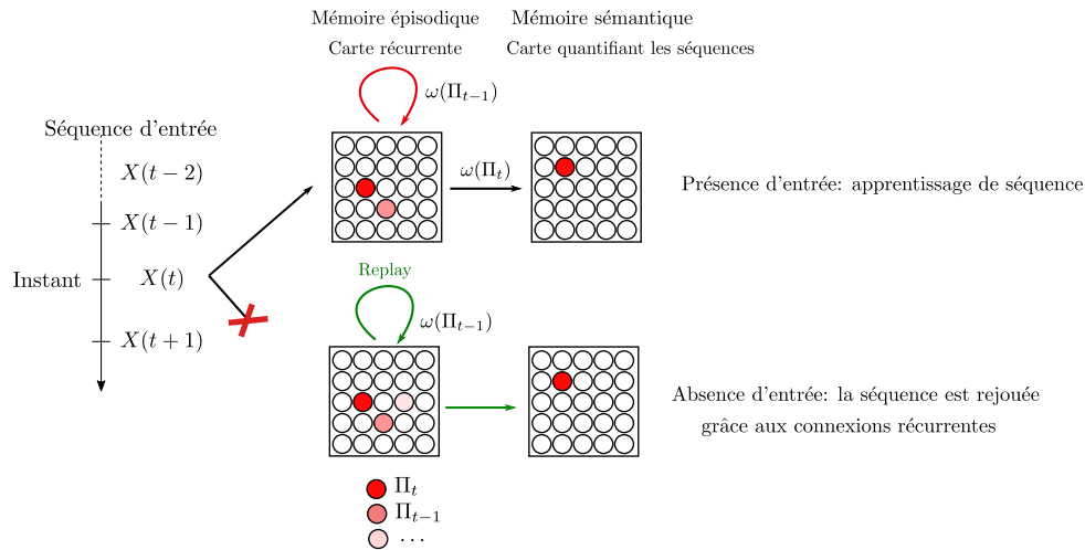
FIGURE 1.20 – Architecture à double mémoire proposée en Parisi et al. 2018 . La couche de mémoire épisodique, permettant la différenciation de séquences, prend en entrée externe un instant de la séquence d'entrée X et en entrée de contexte le poids du BMU de l'instant précédent. La couche de mémoire sémantique est entraînée à partir du poids des BMU de la couche épisodique. Les auteurs ajoutent des conditions de classification supervisant la mise à jour de ces cartes, que nous ne détaillons pas sur ce schéma. Ce modèle est un exemple d'architecture assemblant cartes récurrentes et cartes classiques; il s'agit ici d'un modèle semi-supervisé. Les auteurs utilisent cette architecture dans le cadre de l'apprentissage à long-terme.
