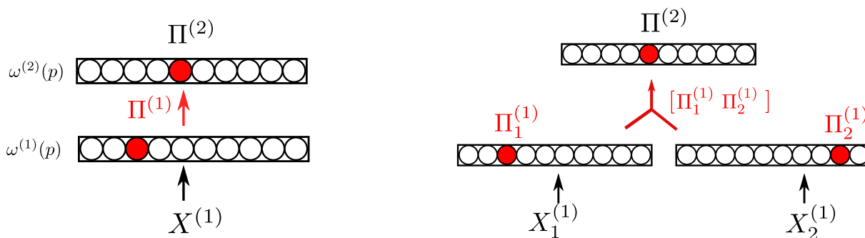
FIGURE 1.10 – Deux exemples d’architectures basées sur HSOM. À gauche, le modèle HSOM original proposé en Lampinen et E. Oja 1992. L’apprentissage des positions du BMU de la première couche par la seconde permet de mieux détecter les ensembles de données présents dans la distribution des X ( clustering ). La deuxième couche est vue comme un niveau plus abstrait que la première. À droite, une version de HSOM comportant plus de cartes proposée en Hagenauer et Helbich 2013 permettant de faire du clustering sur des entrées provenant de deux espaces X_1^{(1)} et X_2^{(1)} . Ces deux espaces sont ici des caractéristiques spatiales et temporelles d’un environnement d’entrée.
