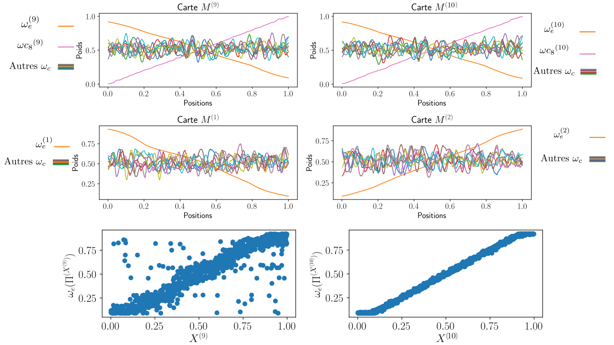
FIGURE 5.29 – En haut, tracé des poids des cartes pour une architecture de 10 cartes toutes connectées. Nous avons ici seulement tracé 4 cartes sur les 10. Les entrées sont toutes indépendantes, sauf les entrées X^{(9)} et X^{(10)} qui sont identiques. Les poids contextuels \omega_{c_8}^{(9)} et \omega_{c_8}^{(10)} correspondent à la connexion entre M^{(9)} et M^{(10)} . Nous remarquons que les poids contextuels ont évolué vers une valeur moyenne autour de 0.5, sauf ceux correspondant aux entrées dépendantes qui se sont dépliés. En bas, nous traçons l'erreur de prédiction de la carte 9 lorsqu'elle ne reçoit pas d'entrée. La prédiction est assez bien réalisée : les connexions contextuelles inutiles perturbent peu l'encodage du modèle.
